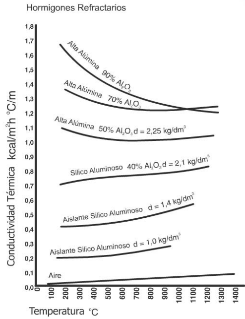
Curva Típica de Conductividad Térmica
